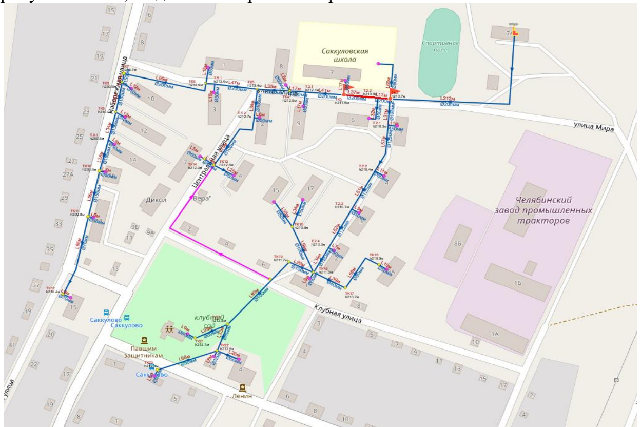
Рисунок 11.6.1. Сценарий развития аварии системы теплоснабжения Котельной п. Саккулово
